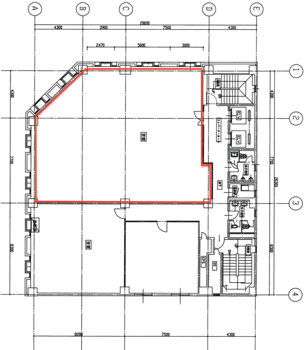
4階平面図
